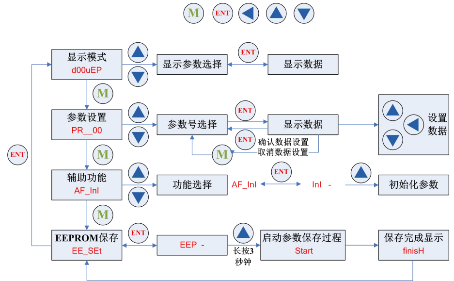
图 5 按键操作流程图
